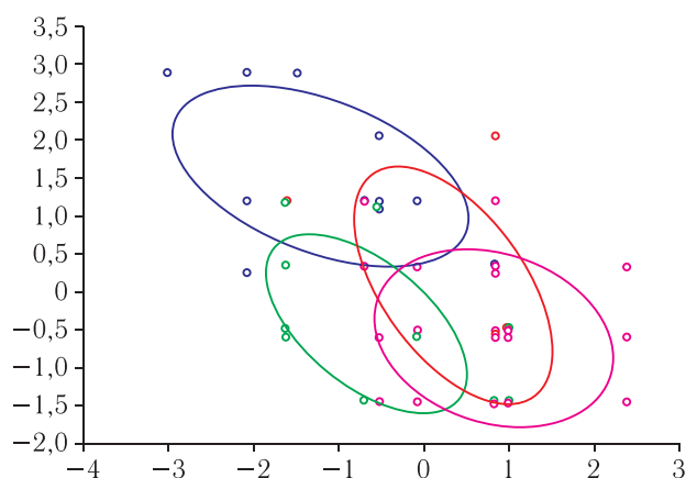
Рис. 8. Двумерная диаграмма дискриминантных функций, классифицирующих некроз и выживаемость: синий эллипс — выжившие без некроза кишки, зеленый эллипс — выжившие с некрозом кишки, красный эллипс — умершие без некроза кишки, розовый эллипс — умершие с некрозом кишки.
